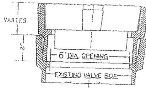
1, 1 1/2, 2, 2 1/2" PAVADJUSTER
