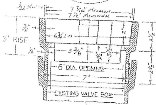
3" PAVADJUSTER
